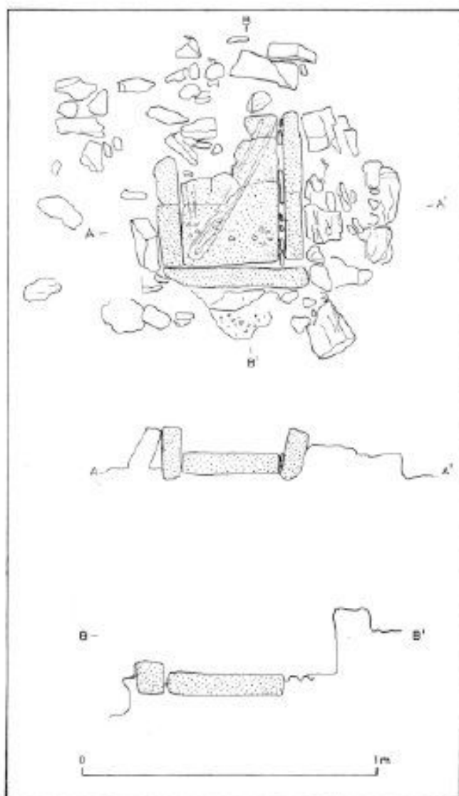
FIG. 4. Planta y secciones de la estructura 20.
