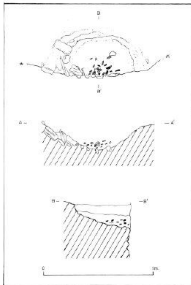
FIG. 6. Planta y secciones de la estructura 22.
