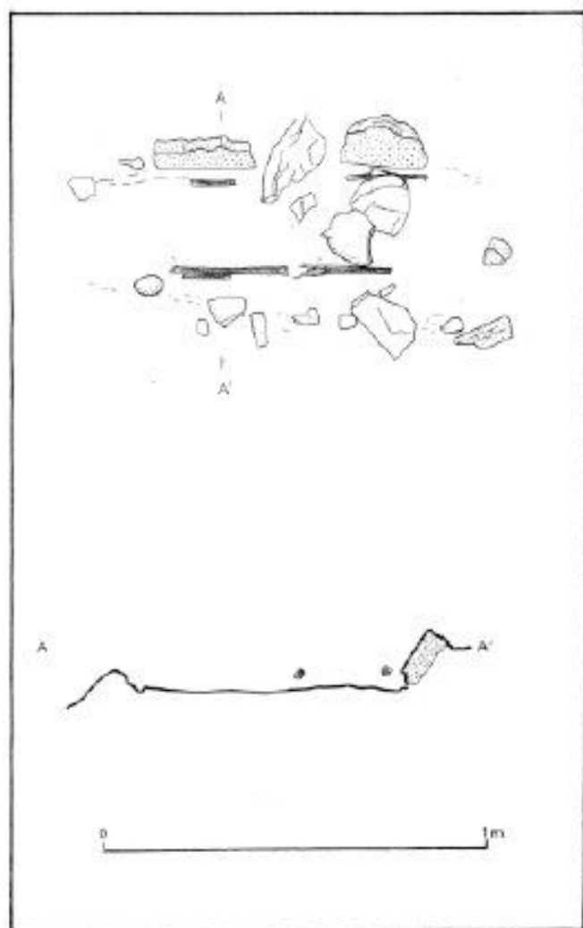
FIG. 3. Planta y secciones de la estructura 18.
